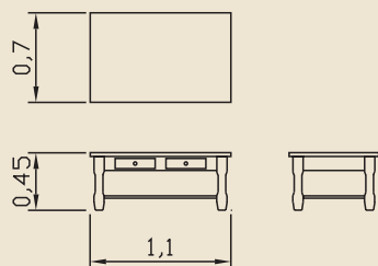
METS 0023 COFFEE 0023 ΜΑΣΙΦ ΤΙΚ 110 x 70 x 45
